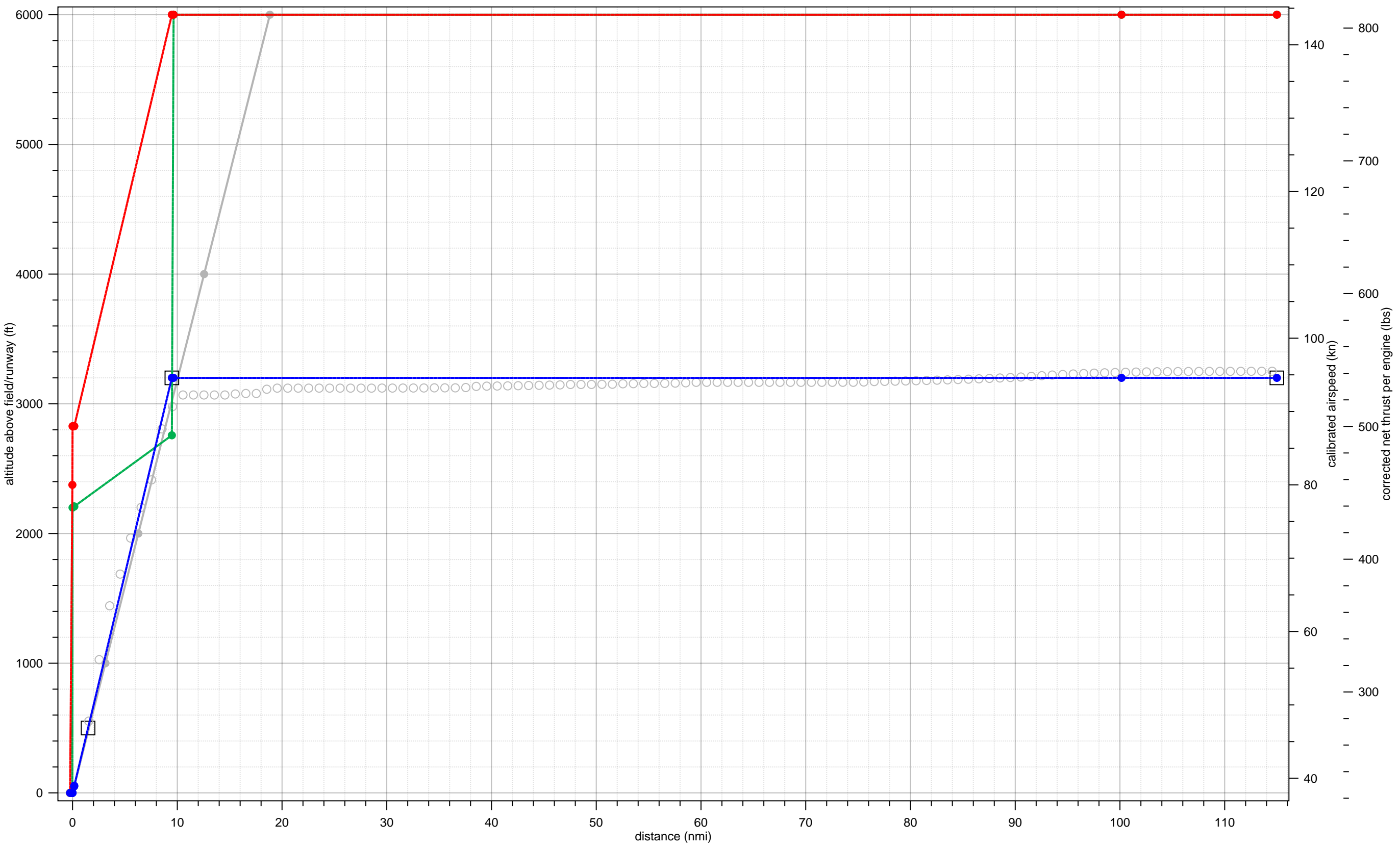
DO228 fit to 13-A-C130-LT-1-3000-50andup-6to15
